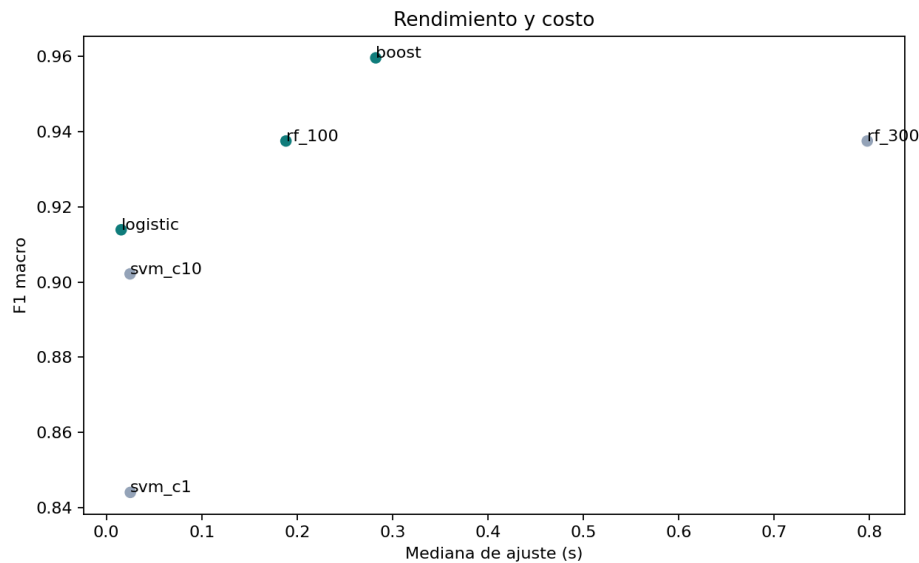
Figura 2. F1-macro frente a mediana de ajuste. En verde, los modelos de la frontera de Pareto.
