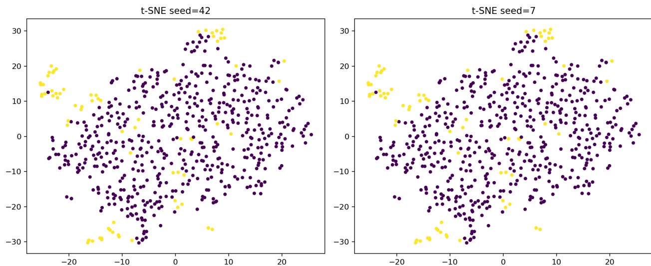
Figura 1. t-SNE con semillas 42 y 7. Morado: donante ( no ); amarillo: enfermo ( si ).
